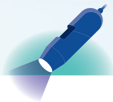
ULTRAVIJOLIČNA (UV)
