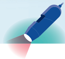
INFRARDEČA (IR)
